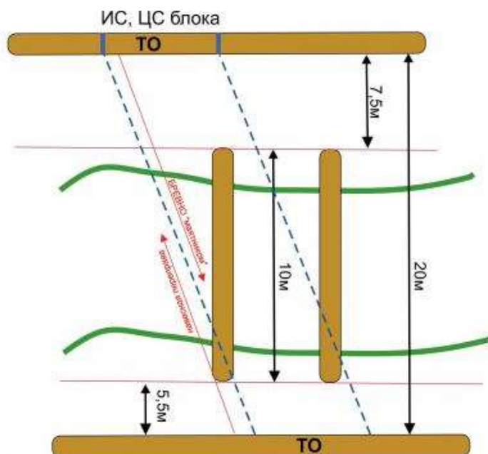
Блок №1. Переправа маятником по бревну - навесная переправа (вид сверху)
