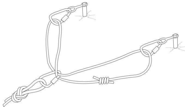
Рисунок 2. Схема блокировки ледобуров с помощью компенсационной петли.
