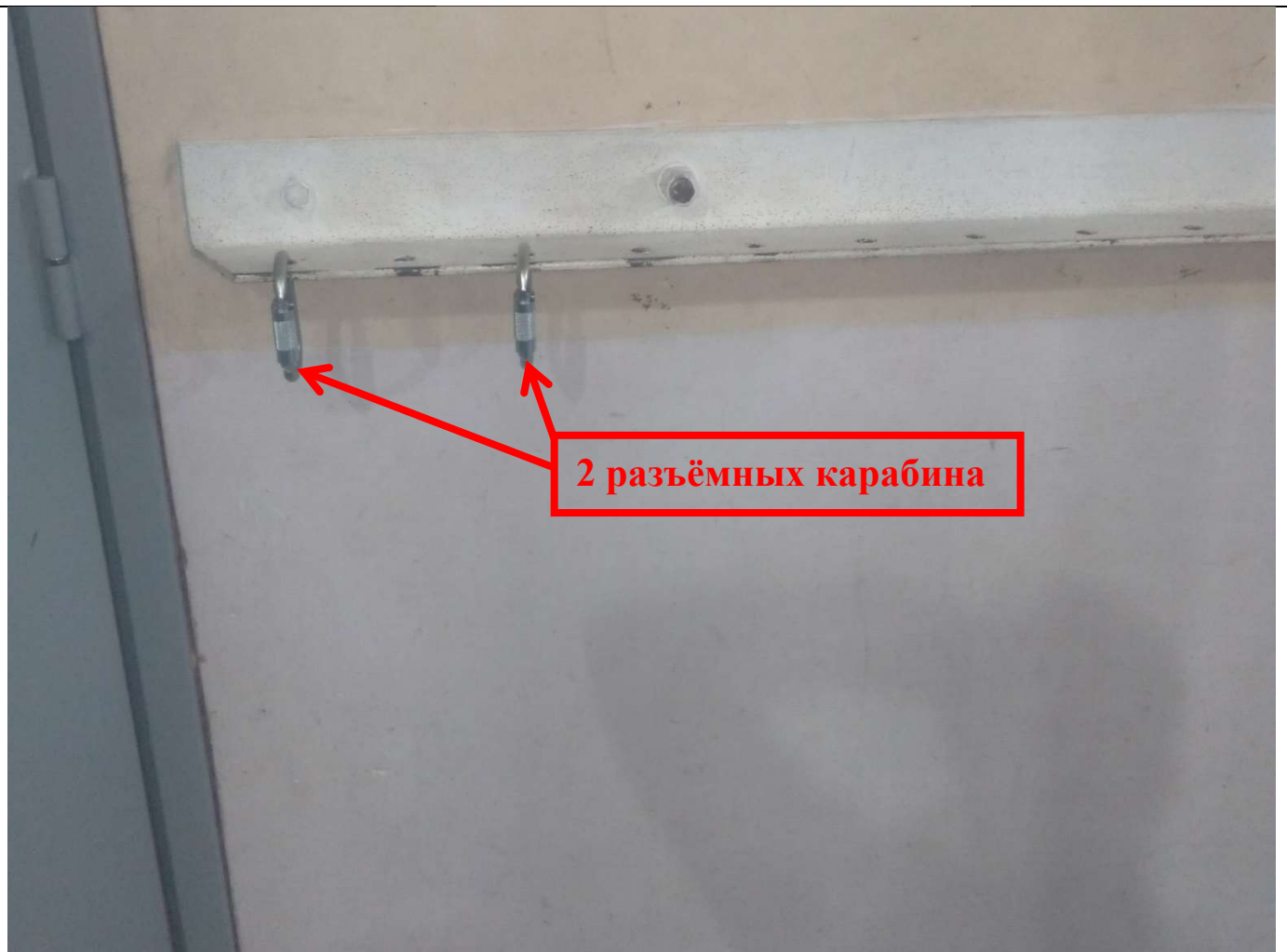
ТО - 7
