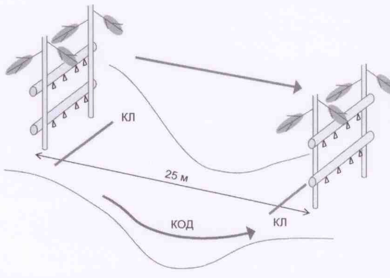
Этап 5. Переправа по параллельным перилам
