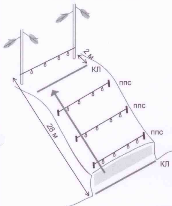
Этап 1. Подъем в кошках с командной страховкой
